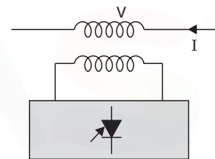
Fig. 21.23 ATCSC.
